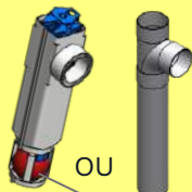
Dispositif de sortie de la décantation primaire
