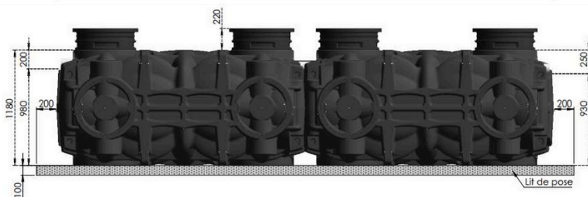
GINETT PE 7EH H et 9EH H
