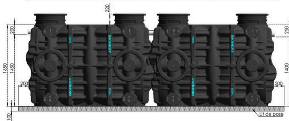
GINETT PE 7EH V et 9EH V
