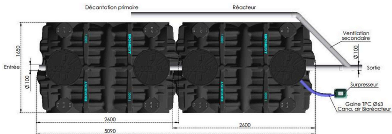
GINETT PE 7EH V et 9EH V
