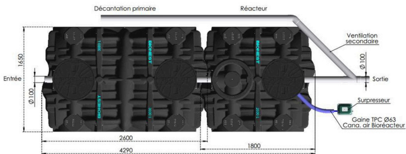
GINETT PE 5EH XL V
