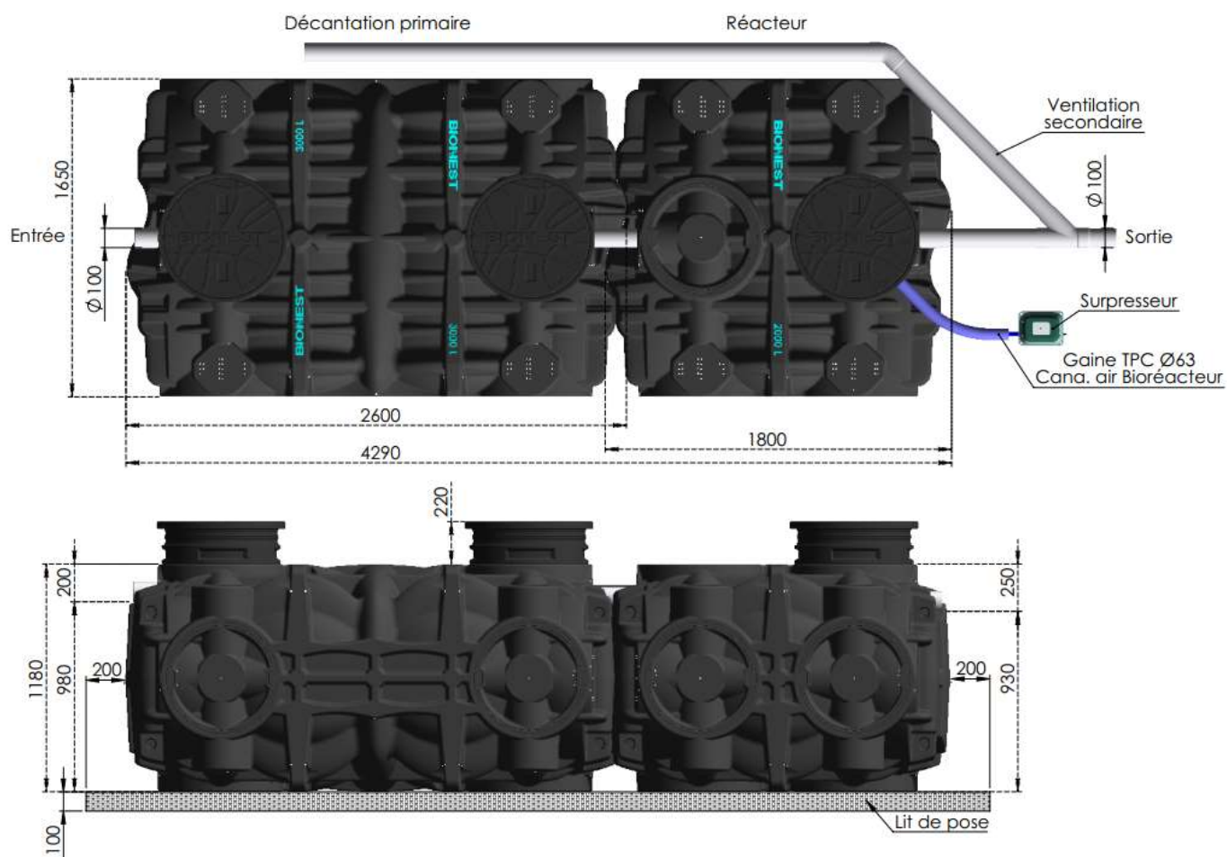
GINETT PE 5EH XL H
