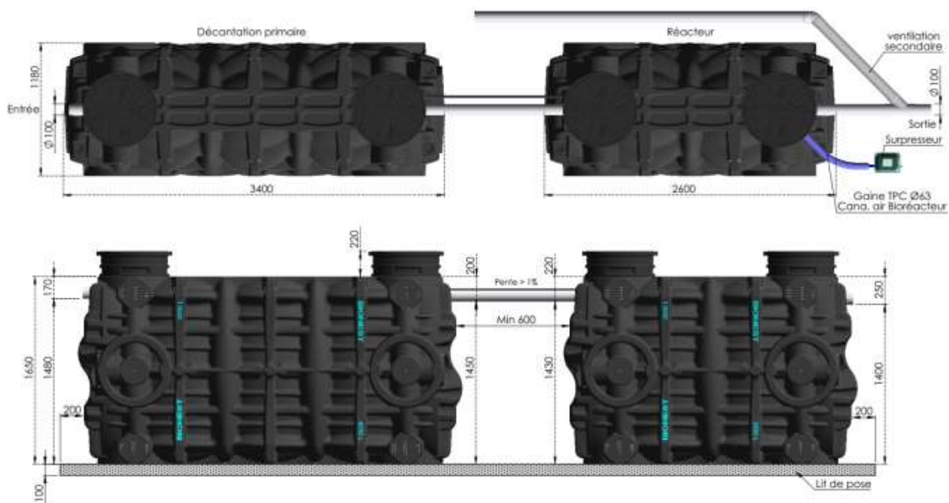
GINETT PE 10EH V
