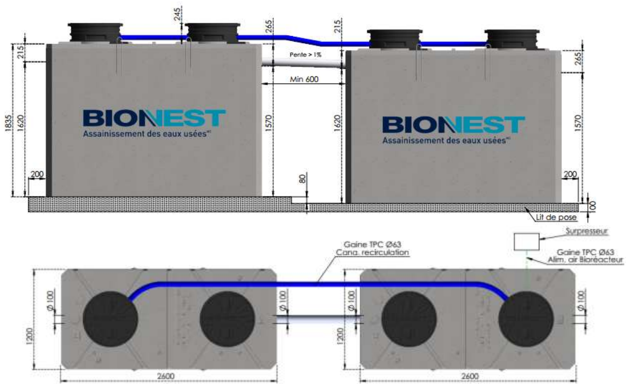
GINETT béton 13EH
