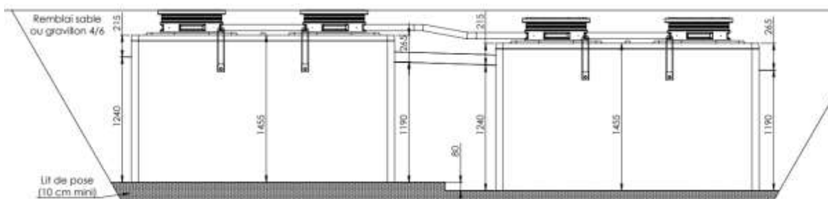
Figure 24 : Lit de pose (ex : GINETT béton 7EH Bic)
