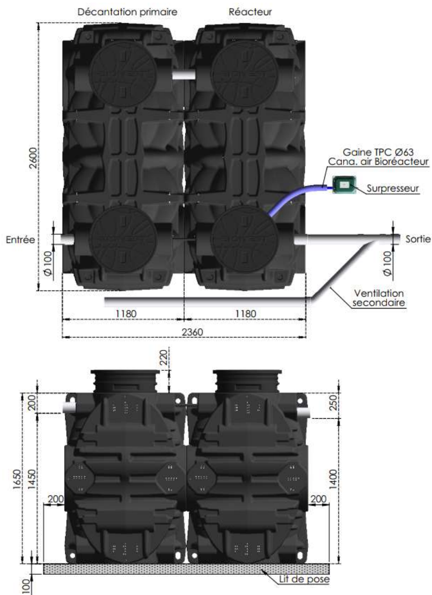
GINETT PE 7EH Pack et 9EH Pack
