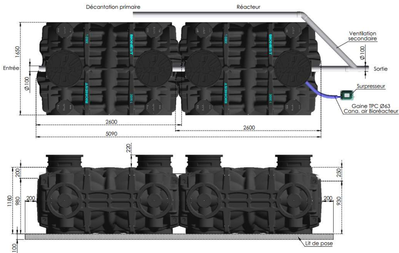
GINETT PE 7EH H et 9EH H
