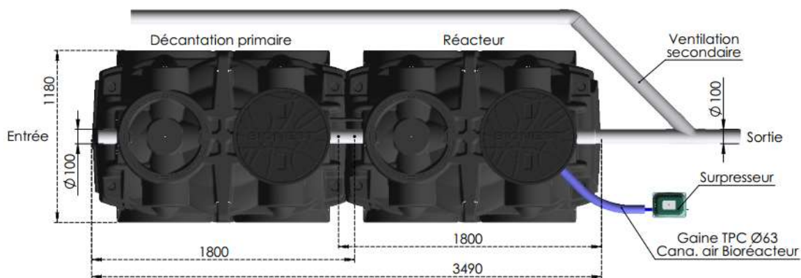
GINETT PE 4EH Pack
