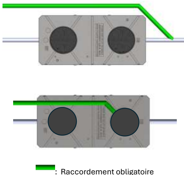
Figure 37: Piquages de la ventilation secondaire sur les modèles monocuve
