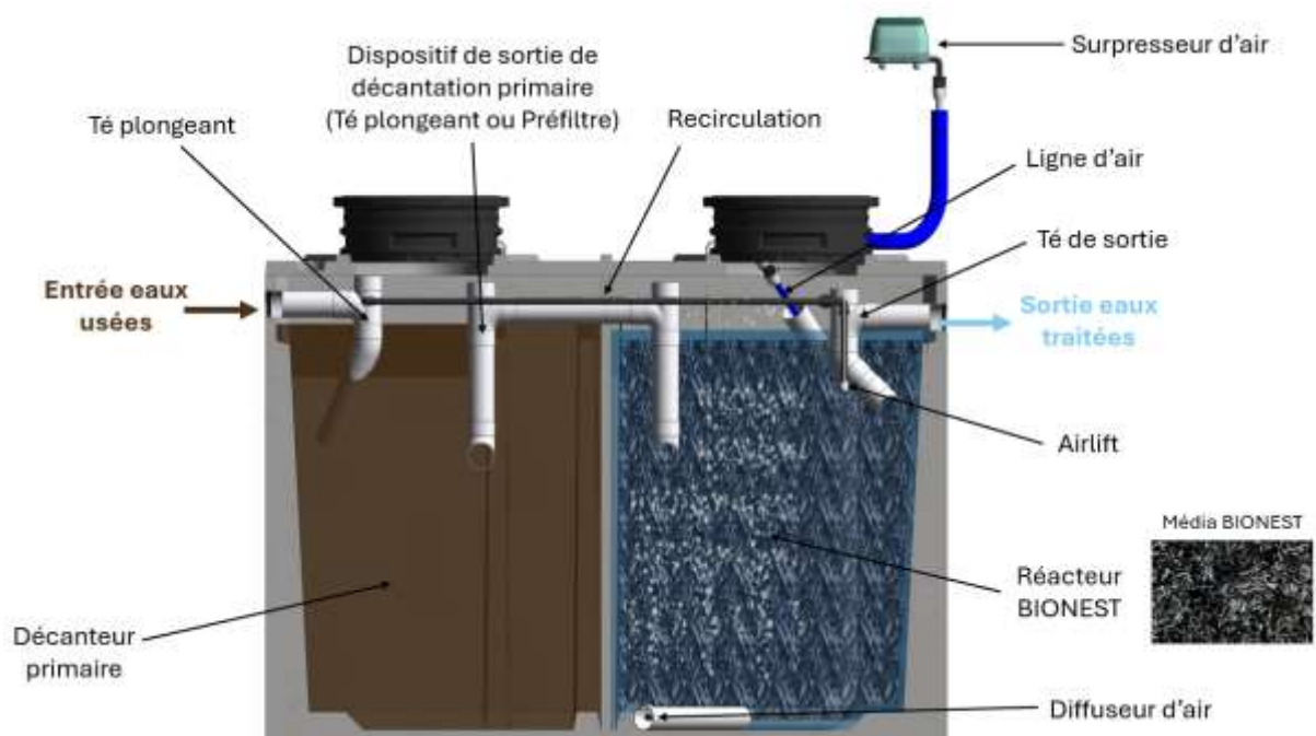
Figure 2 : Schéma de principe d'une filière GINETT monocuve béton
